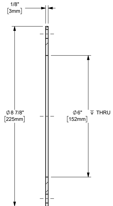
SECTION A-A
