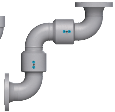
150# ASA flange x 150# ASA flange
